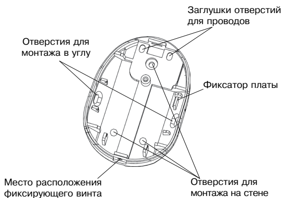
Рисунок 2 – Основание извещателя
