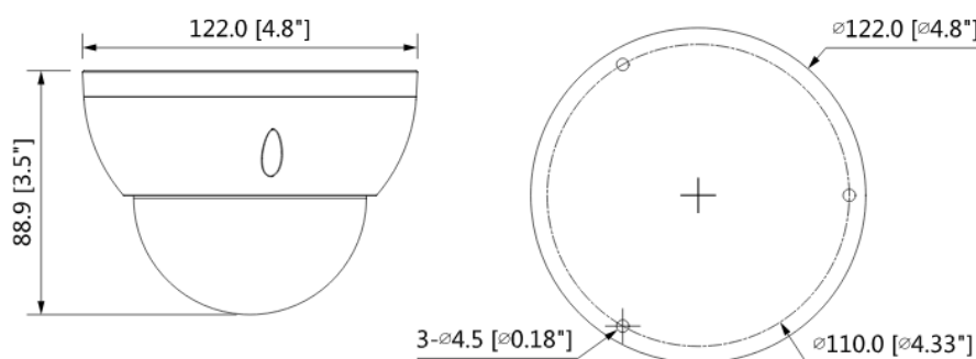
Рисунок 5.1 – Габаритные размеры видеокамеры
