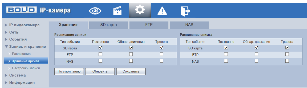
Рисунок 7.100 — Вкладка «Хранение»
