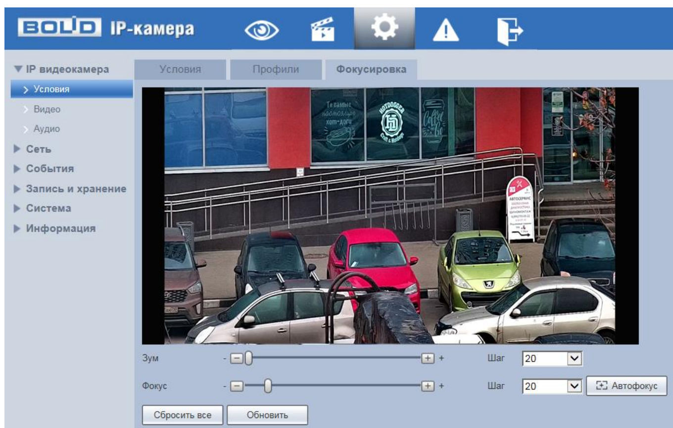
Рисунок 7.37 — Вкладка «Фокусировка»
