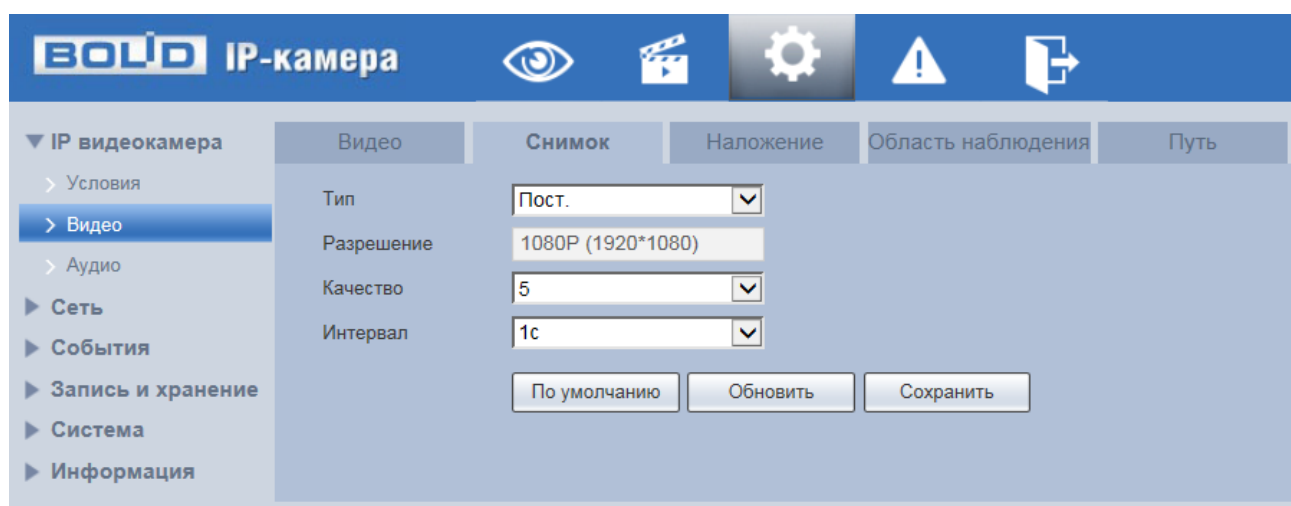
Рисунок 7.40 — Вкладка «Снимок»
