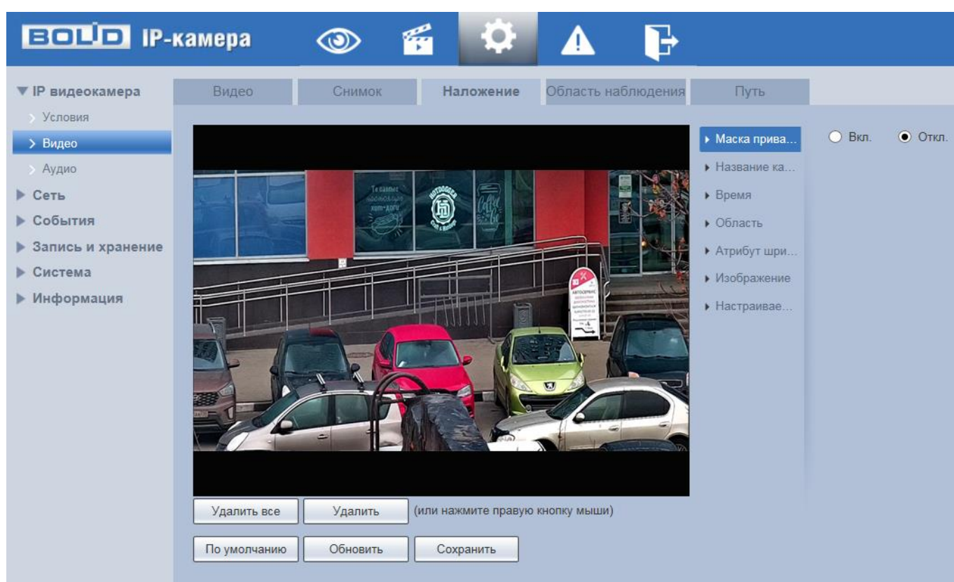
Рисунок 7.41 — Вкладка «Наложение»
