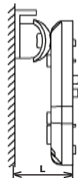
Рисунок 2 - Основание извещателя и кронштейн
