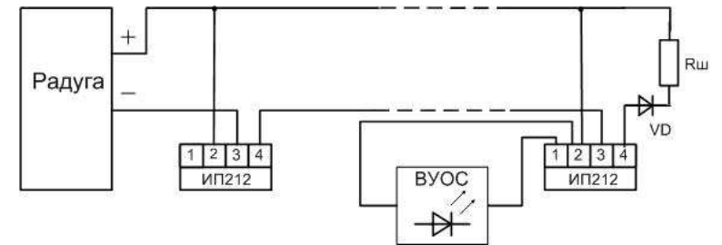
Рисунок А.3 Схема подключения извещателей к прибору ПС-4
