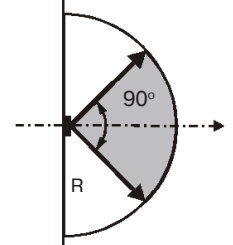
Рисунок 2 – Диаграмма зоны обнаружения АК канала
