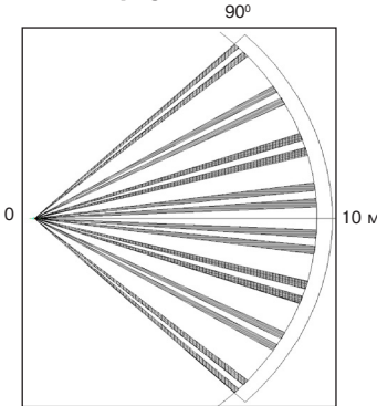
Рисунок 1 – Диаграмма зоны обнаружения ИК канала
