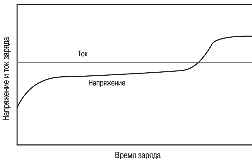
Рис. 4 График заряда постоянным током.
